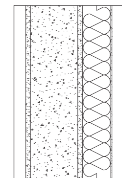
Dettaglio 04 Parete esterna vano scala
