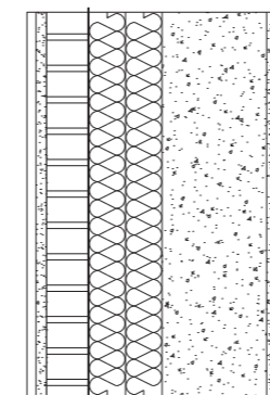
Dettaglio 03 Parete verso vano ascensore
