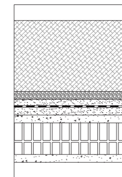
Dettaglio 06 Solaio verso giardino
