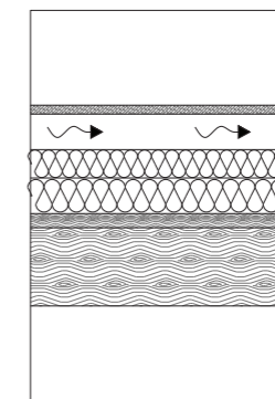
Dettaglio 04 Solaio copertura inclinata
