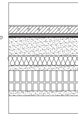
Dettaglio 02 Solaio verso piano interrato
